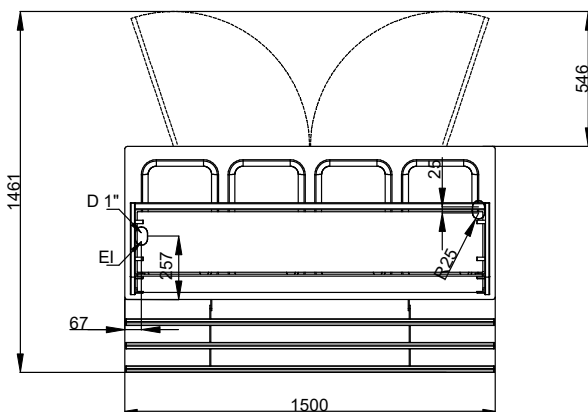
Dessus
